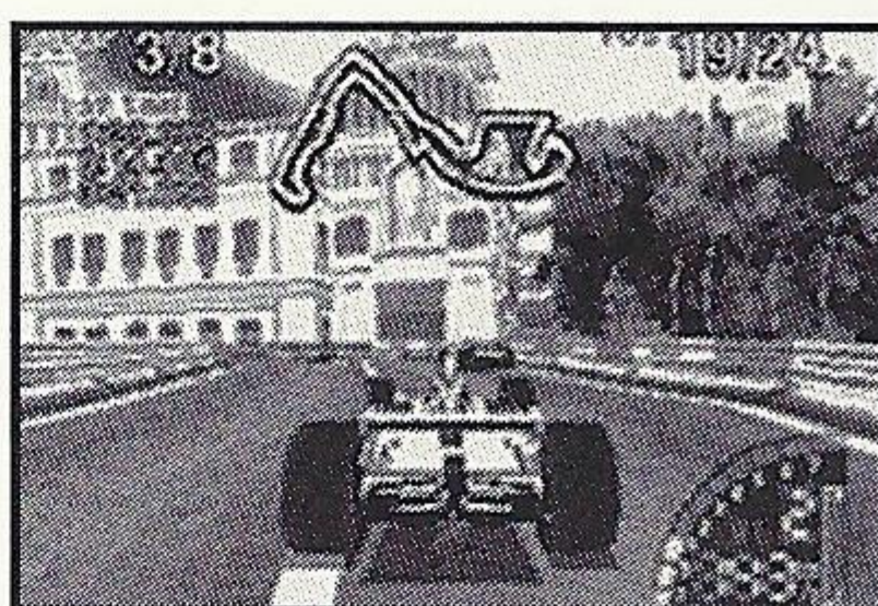
Monte Carlo
